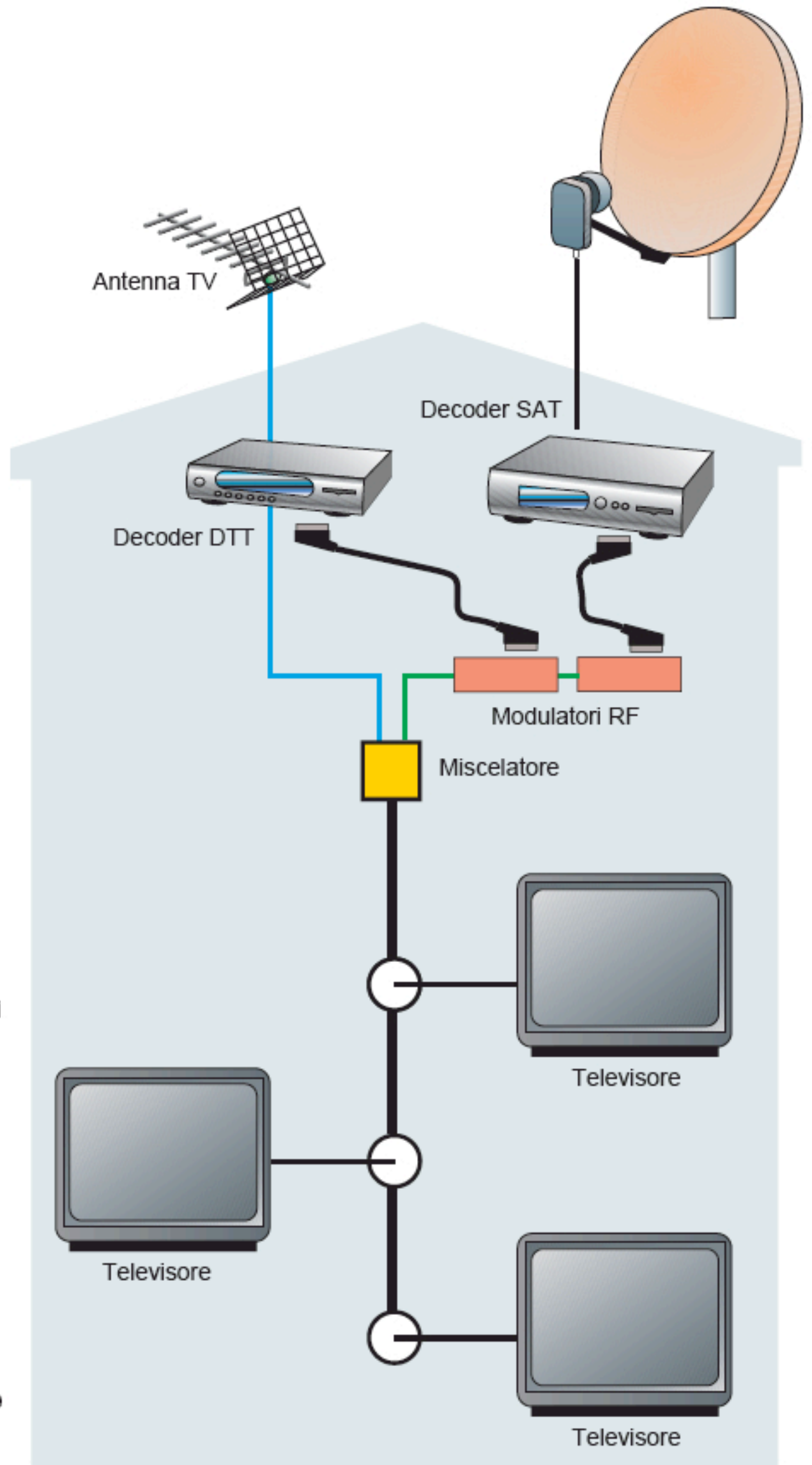
Figura 6. Per portare i programmi Tv digitali a tutti i televisori di casa, impiegando un solo decoder Sat e DTT, si possono usare due modulatori RF stereo collegati in testa all'impianto di distribuzione dell'appartamento. Ovviamente tutti vedranno gli stessi programmi e sarà necessario aggiungere alcuni ripetitori di telecomando
